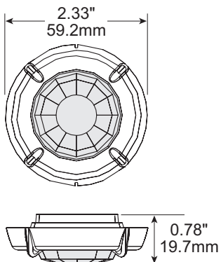
FSP-L2 dimensions
