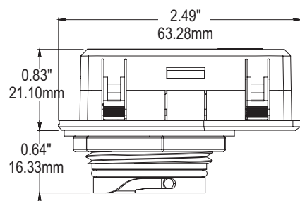
FSP-202 dimensions
